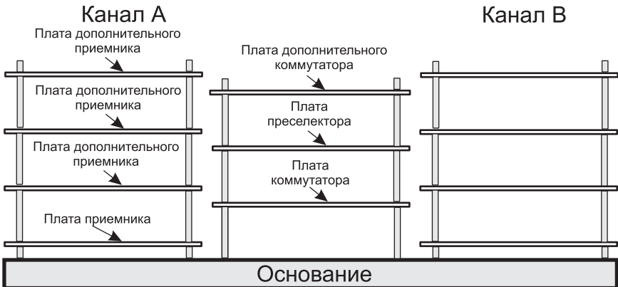
Вариант размещения восьми приемников (четыре частотные литеры)
