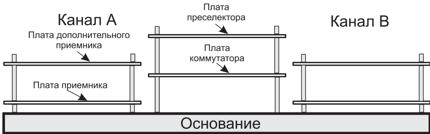
Вариант размещения четырех приемников (две частотные литеры)
